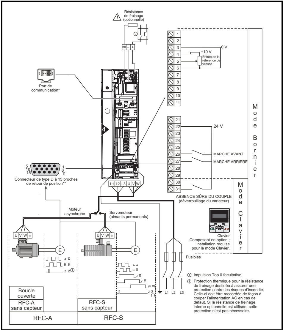
Figure 6-1 Connexions minimales pour la mise en marche du moteur dans tous les modes de fonctionnement (taille 4 illustrée)
