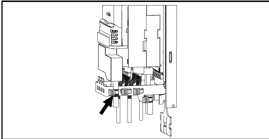
Figure 3-4 Mise à la terre des blindages des câbles de signal à l'aide de l'étrier de blindage
