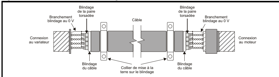
Figure 3-5 Raccordements du blindage du câble de retour
