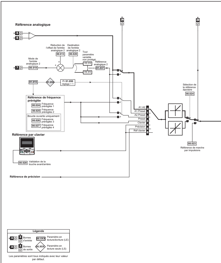
Figure 5-1 Schéma logique du menu 0
